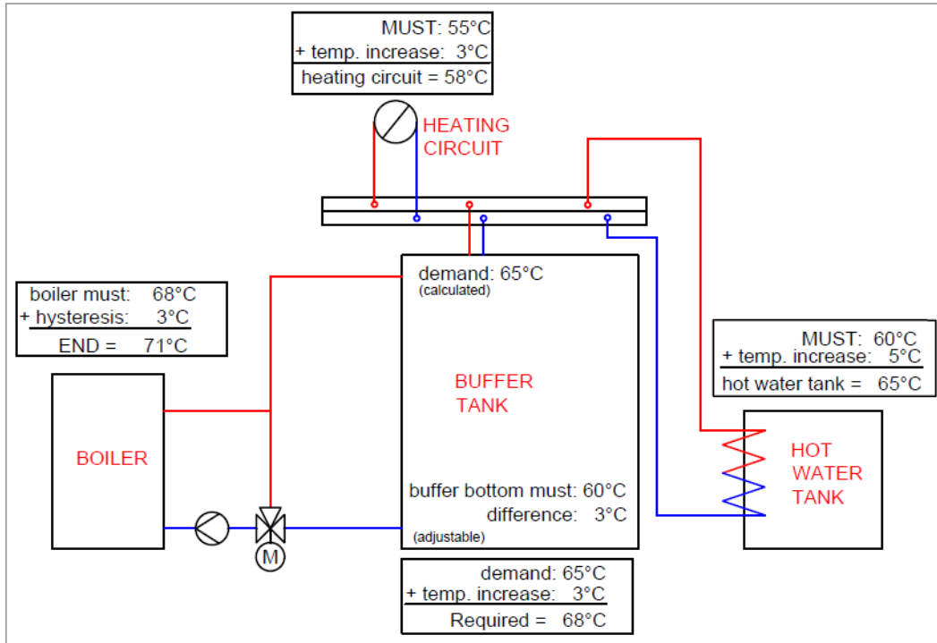
Figura 8.2: Ejemplo gestión temperatura con depósito de inercia y sin diferencia
